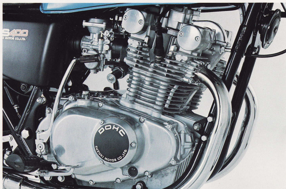
● 2 cylindre, 2 overliggende knastaksler, 6 gear — lynhurtig acceleration og smidig, kultiveret motorgang.
