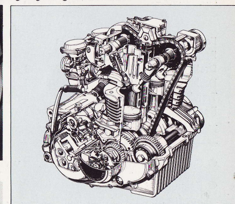
● Kædetræk til to overliggende knastaksler. Automatisk justering — altid korrekt kædespænding. El-start. Servicevenlig motorkonstruktion.
